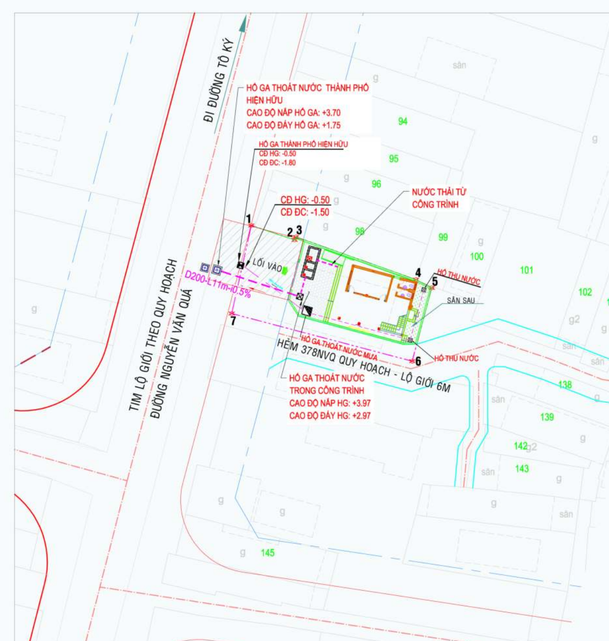
BẢN ĐỒ QUY HOẠCH HỆ THỐNG THOÁT NƯỚC
