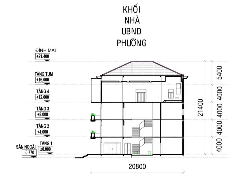
MẶT CẮT A-A TỶ LỆ 1/500
