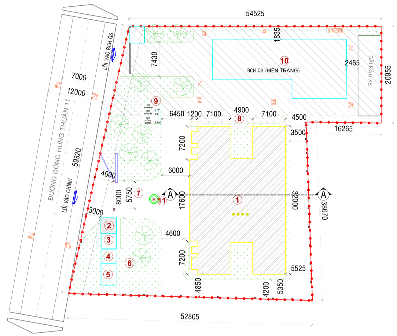
MẶT BẰNG TỔ CHỨC KHÔNG GIAN KIẾN TRÚC CẢNH QUAN TỶ LỆ 1/500
