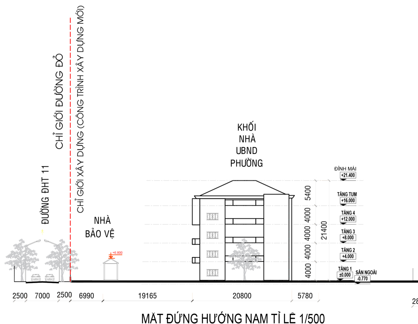
MẶT ĐỨNG HƯỚNG NAM TỶ LỆ 1/500
