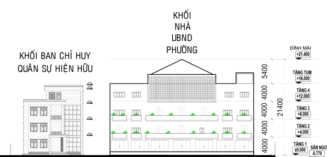
MẶT ĐỨNG HƯỚNG TÂY TỶ LỆ 1/500
