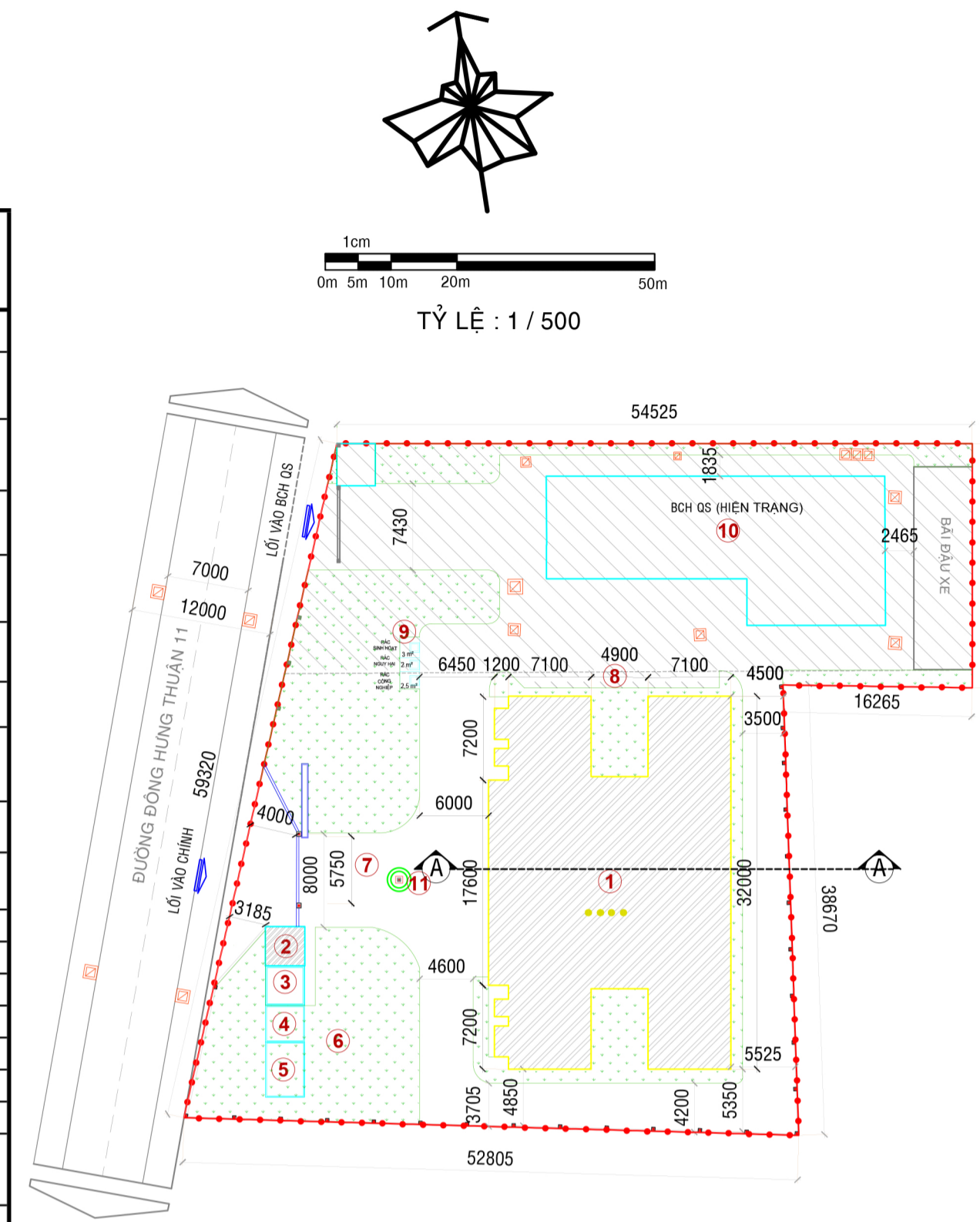
MẶT BẰNG TỔNG THỂ - TỶ LỆ 1/500
