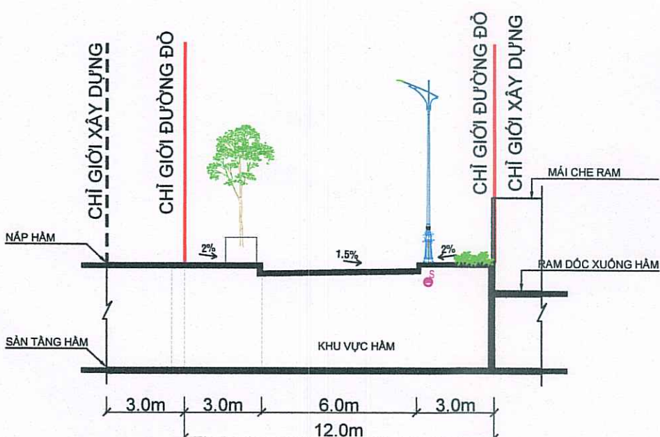
MẶT CÁT 2-2 TỶ LỆ 1/200
